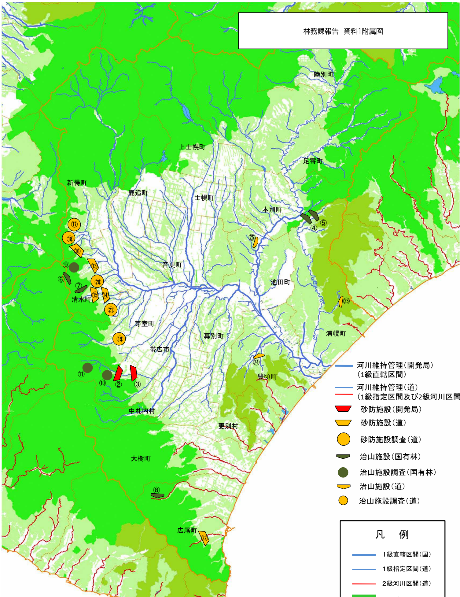
流木発生抑制に係る事業位置図 令和2年度 実績
